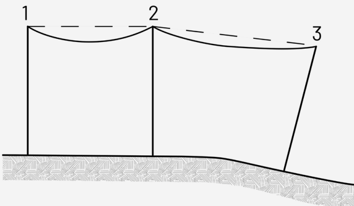
Rys. 3. Schemat wpływu przejścia niecki na sekcje linii elektroenergetycznej (b)
