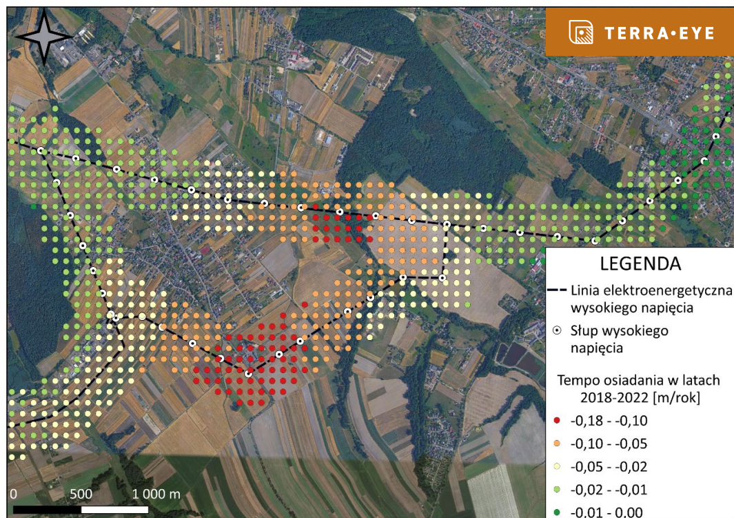
Rys. 5. Prezentacja tempa deformacji podłoża wzdłuż linii elektroenergetycznej.
