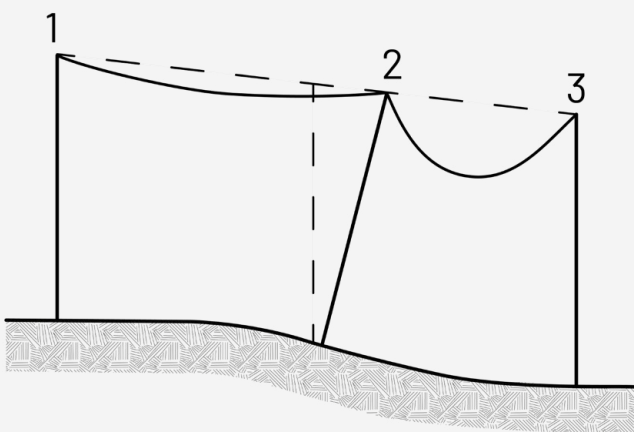
Rys. 4. Schemat wpływu przejścia niecki na sekcje linii elektroenergetycznej (c)
